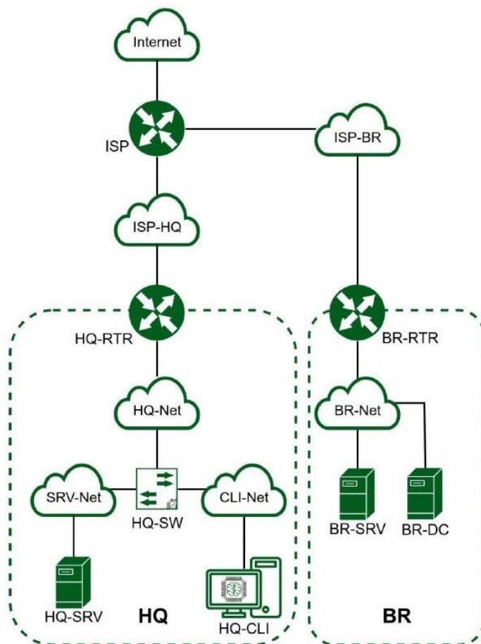
Рисунок 3. Топология сети
