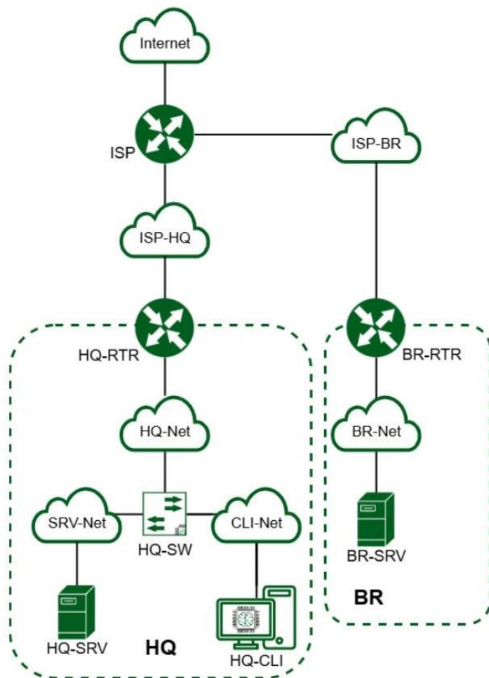
Рисунок 2. Топология сети
