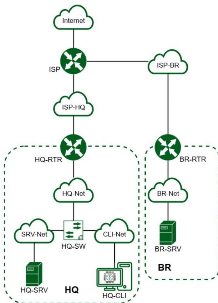
Рисунок 1. Топология сети
