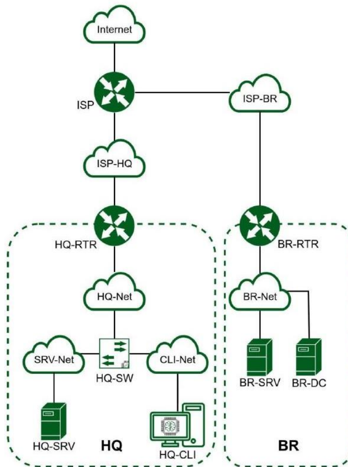
Рисунок 3. Топология сети
