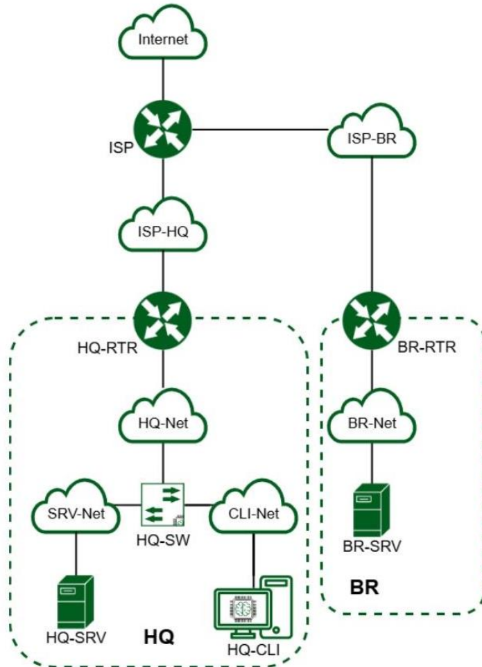
Рисунок 2. Топология сети
